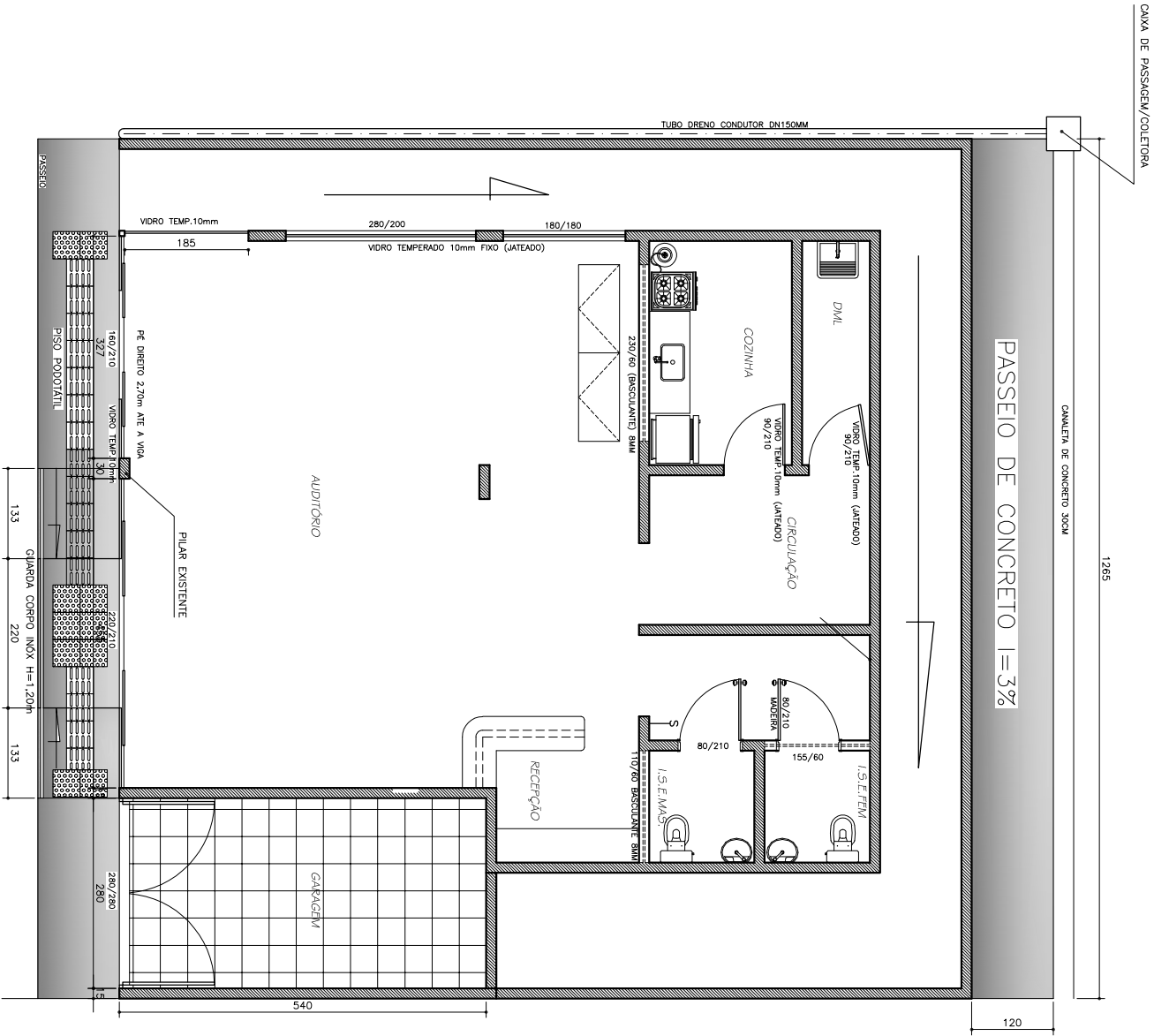
Planta
